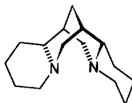
1 : (-)-sparteine
